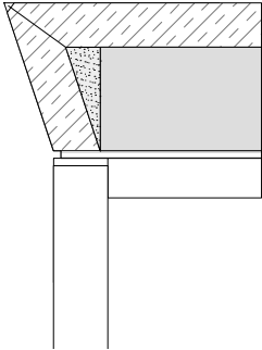
DETAIL SCHUIN OMGEZETTE RAND WERKBLAD
