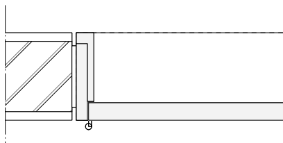
DOORSNEDE VERDIEPT LIGGEND KOZIJN
